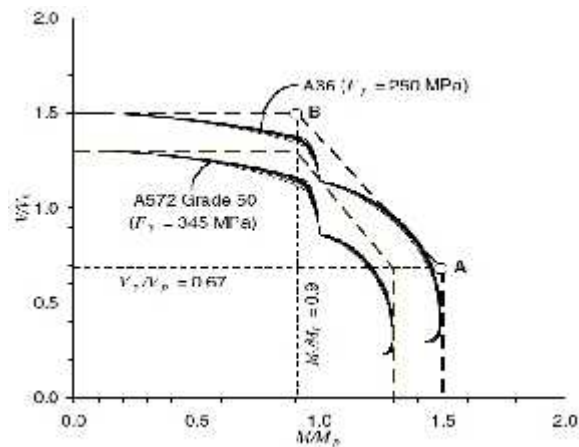
Gambar 2. Diagram interaksi geser-lentur untuk 13 balok tampang W dari AISC untuk baja A36 dan A572 [2]
