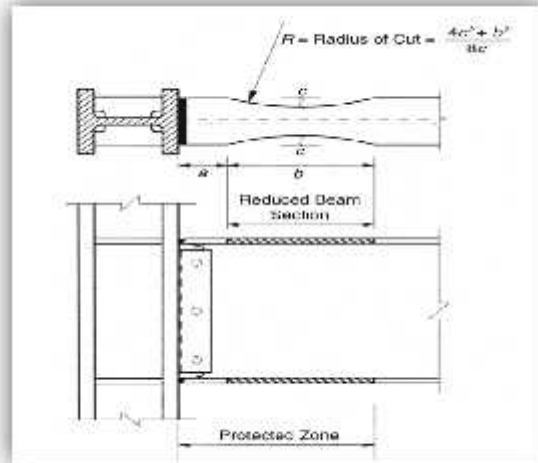
Gambar 1. Detil sambungan RBS
