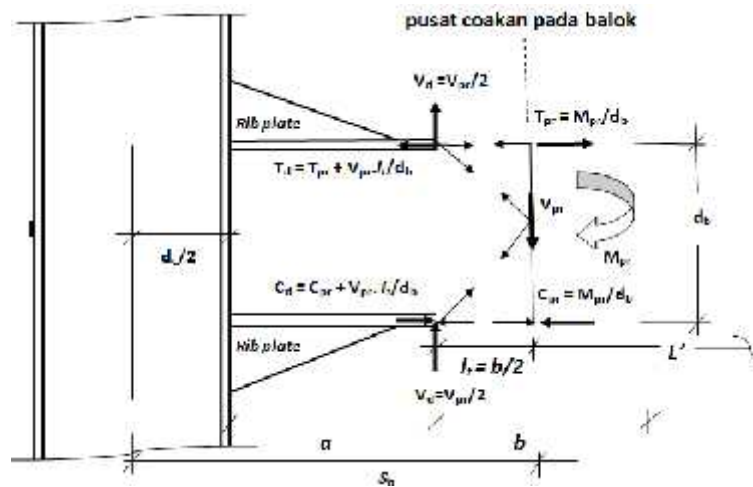
Gambar 6. Truss analogy model pada sambungan RBS
