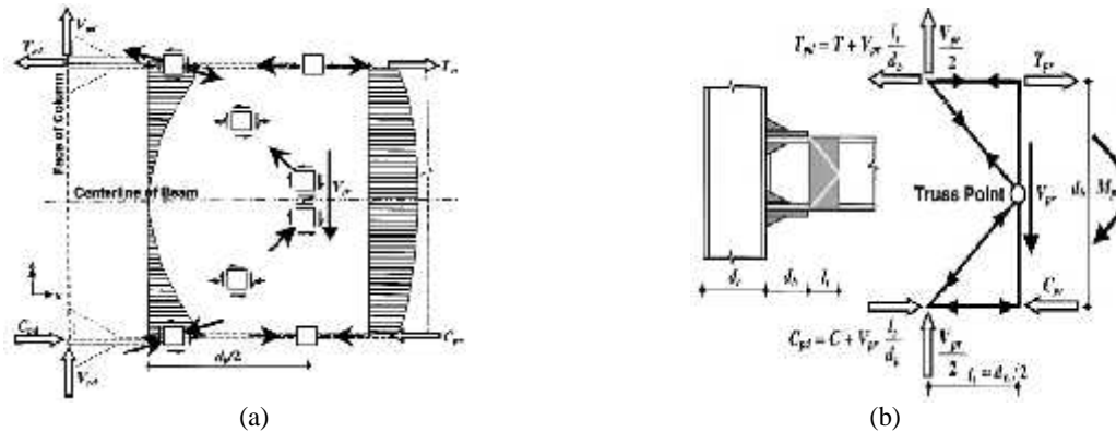
Gambar 5. (a) Arah-arrah tegangan utama maksimum; (b) Pertemuan balok-kolom yang menunjukkan lokasi dan konfigurasi dari improved truss model , dan aliran gaya-gaya yang dipakai untuk merancang sambungan[3]
