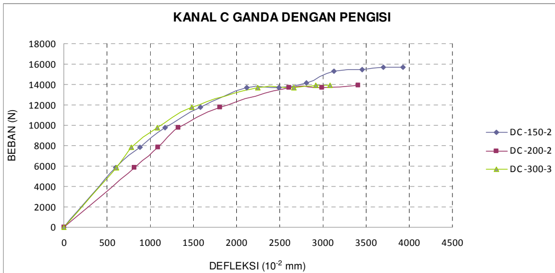
Gambar 10. Perbandingan balok kanal C dengan pengisi
