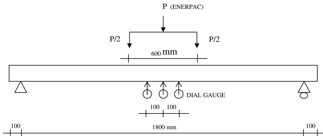
Gambar 3.a. Set up benda uji.
