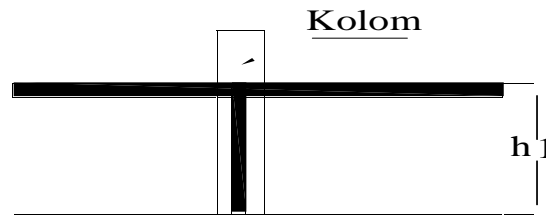
Gambar 5. Perletakan kolom
