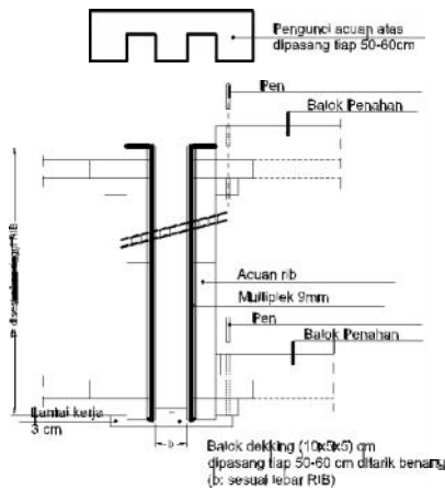
Gambar 8. Potongan A-A
