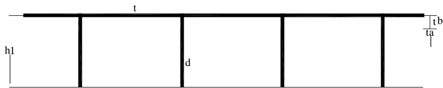
Gambar 3. Bentuk plat pipih menerus dengan rib-rib dibawahnya
