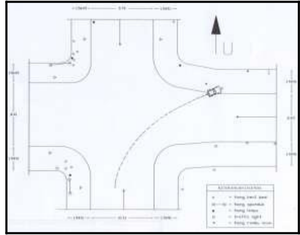
Gambar 7. Skenario I kemungkinan manuver kendaraan menabrak tiang traffic light lengan timur
