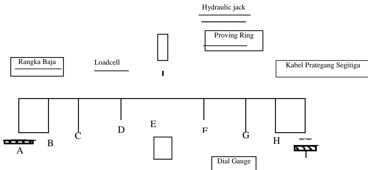
Gambar 3. Skema pembebanan
